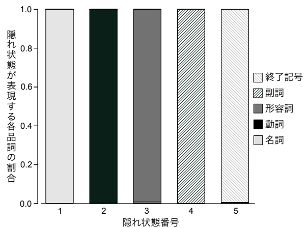
(b) 隠れ状態数 5
