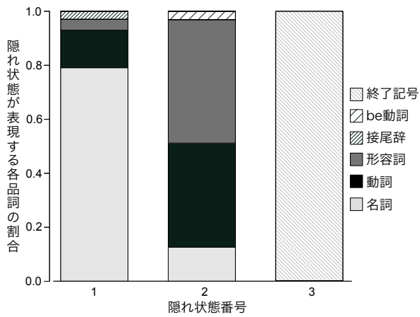
(a) 隠れ状態数 3
