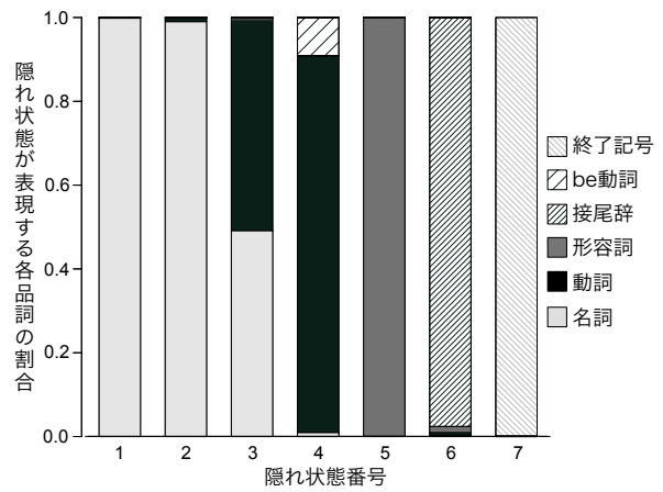
(b) 隠れ状態数 7
