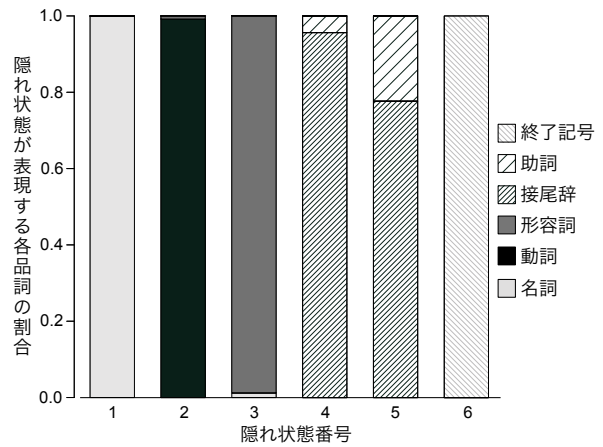
(b) 隠れ状態数 6
